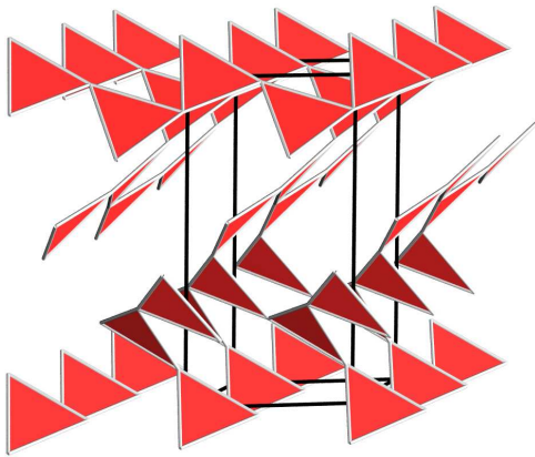
\alpha - B_2O_3
