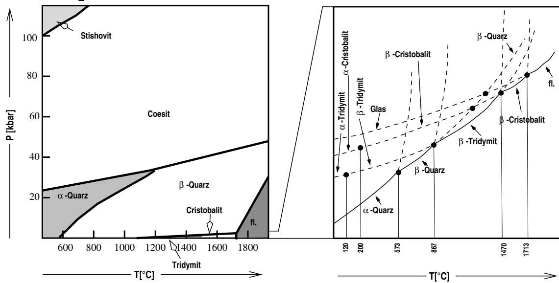
p-T-Phasendiagramm von SiO_2
