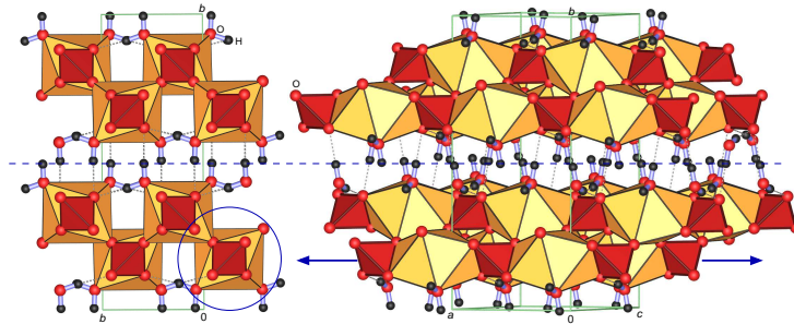
Kristallstruktur von Gips ( \text{CaSO}_4 \cdot 2\text{H}_2\text{O} )
