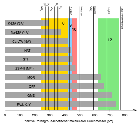
Porenabmessungen und mögliche Gäste
