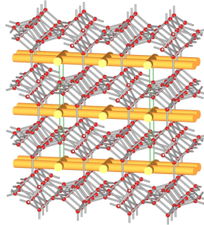
Heulandit (HEU) 9
