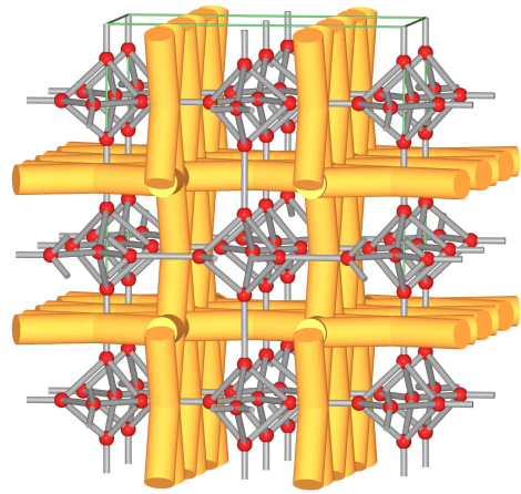
Natrolith (NAT) 12 (sowie 3, 4)
