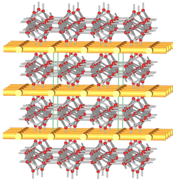
Stilbit (STI) 8
