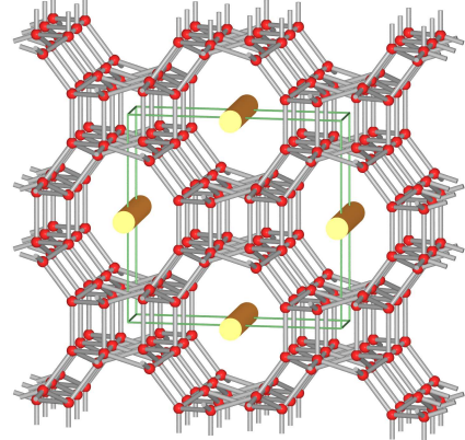
Laumontit (LAU) 6
