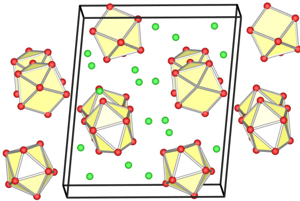
\text{K}_4\text{Sn}_9
