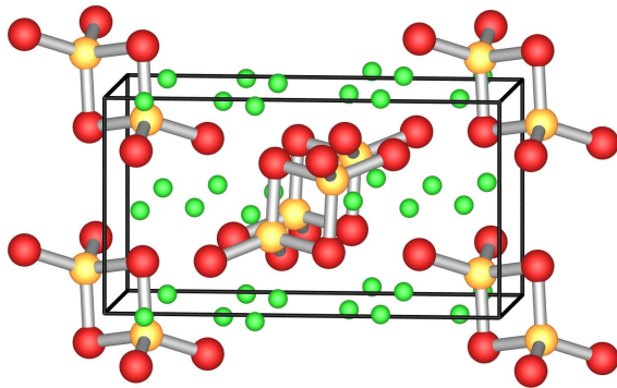
\text{Na}_6\text{Ga}_2\text{Se}_6
