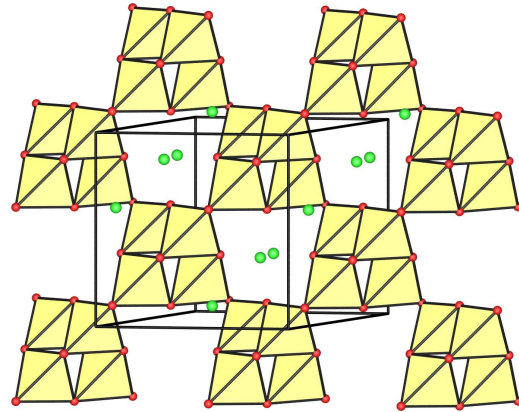
\text{NaAlSe}_2
