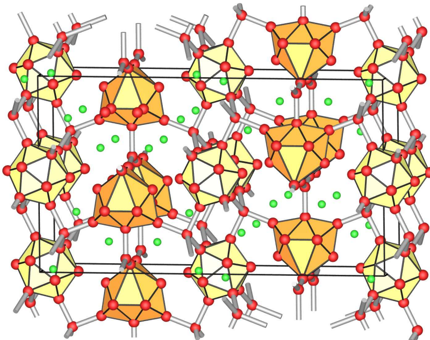
\text{K}_3\text{Ga}_{13}
